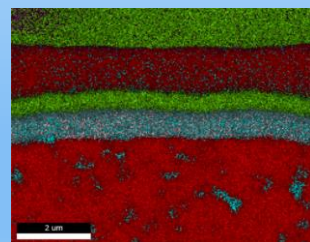
多層膜の元素マッピング
