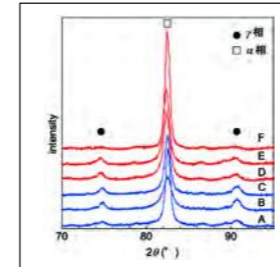
試験後SUS304材のXRDパターン
