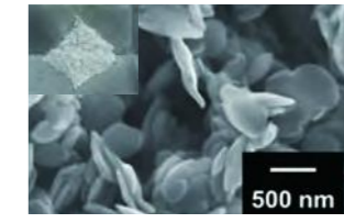
FE-SEMで観察した吸着材原料 (ハイドラタルサイト粉末)
