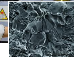
鉄鋼材料破面のSEM像
