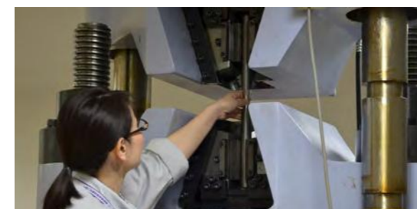
材料試験機による引張試験
