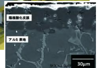
アルミの陽極酸化処理断面のSEM像
