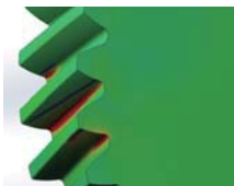
FEMによる応力解析結果。「はすば歯車」のような複雑な形状の製品に対してもFEMを用いれば応力や変位を計算することができます。
