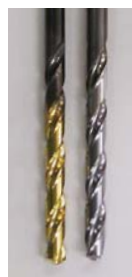
左:窒化チタンコーティング 右:コーティングなし
