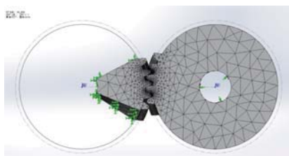
「はすば歯車対」をかみ合わせた場合のFEMによる応力解析モデル
